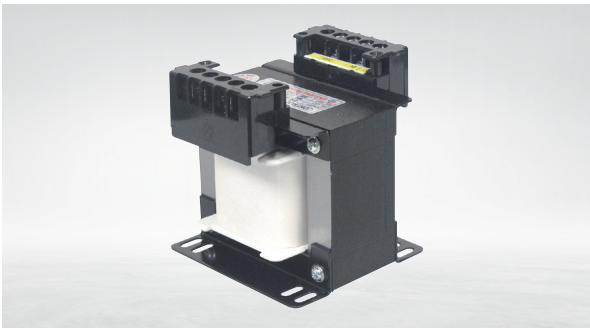
■ SS1 - TSACCS_Auto Trans. CU (50/60Hz)
